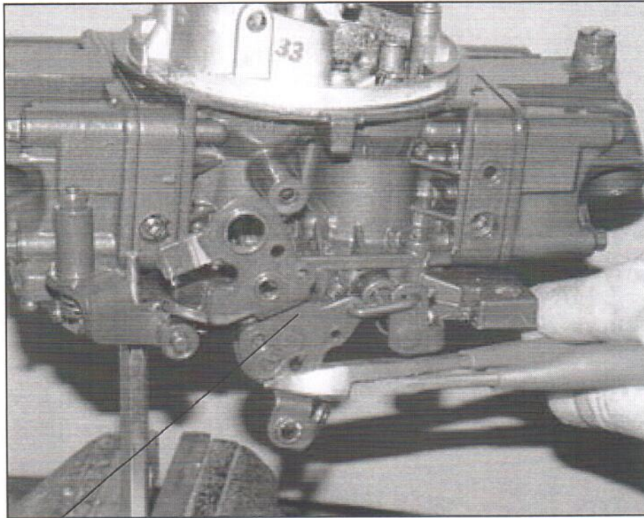
FIGURE F1 CARB LINKAGE MODIFICATION
